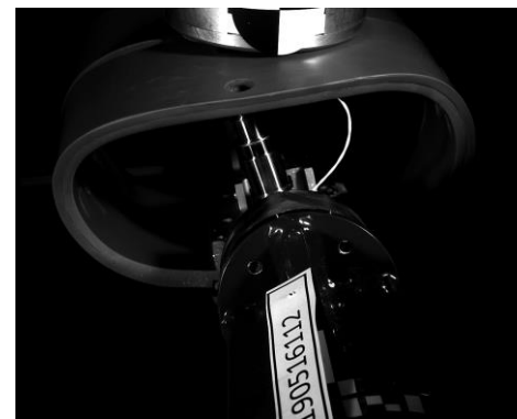
Oblique ribcage tests
